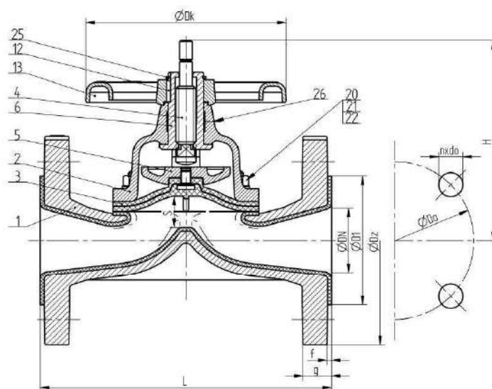
Wymiary przyłączeniowe zaworów membranowych
